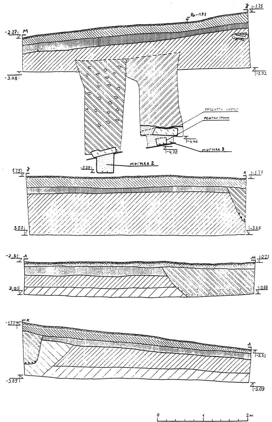
Рис. 23. Некрополь Джург-оба. Стратиграфія стінок м-д суміщених з розрізами могили №2 та могили №3, з-к, л-м, к-л.
