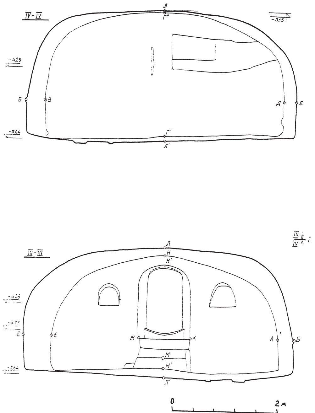
Рис. 7. Некрополь Джург-оба. Розріз по лінії IV-VI суміщеної з фасадом північної стіни. Розріз по лінії III-III суміщеної з фасом південної стіни.
