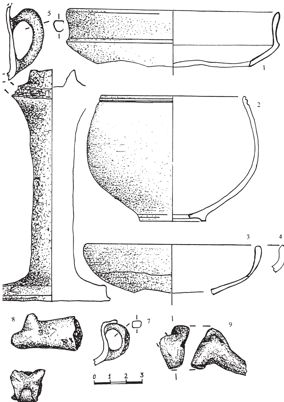
Рис. 10. Некрополь Джург-оба. Матеріал з заповнення поховальної камери склепу №4. 1-4 – червонолакова кераміка. 5-7 – ліпна кераміка. 8-9 – ліпні зооморфні фігурки.
