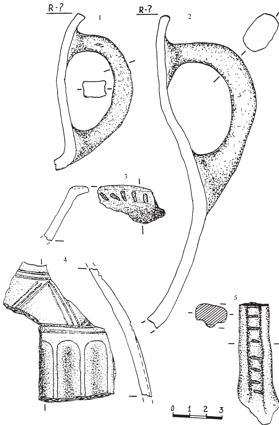
Рис. 18. Некрополь Джург-оба. Матеріал із заповнення переддросної ями склепу №7. 1-5 – фрагменти ліпної кераміки
