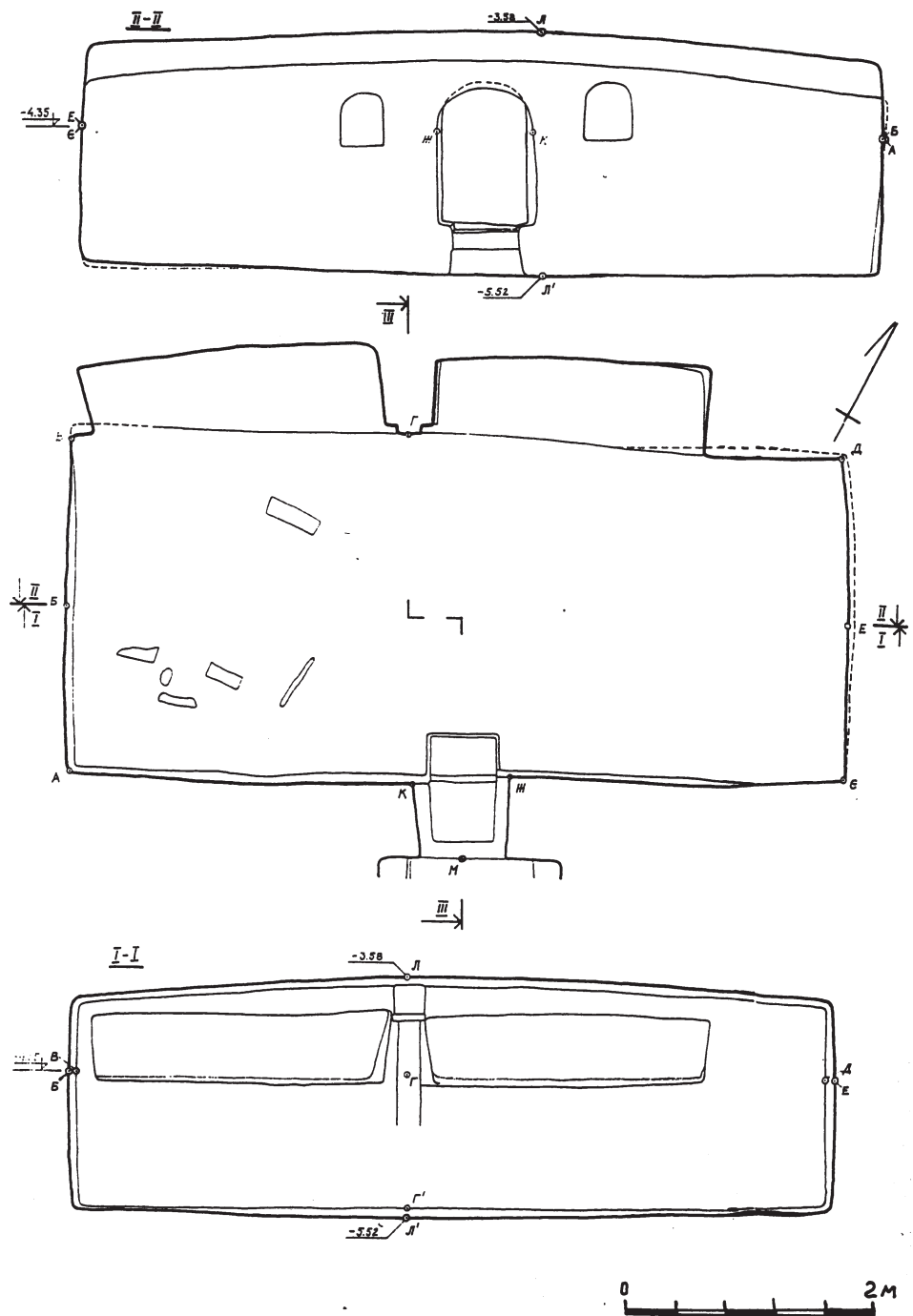
Рис. 15. Некрополь Джург-оба. План поховальної камери склепу №7. Розріз по лінії I-I, суміщений з фасадом північної стіни. Розріз по лінії II-II, суміщений з фасадом південної стіни.
