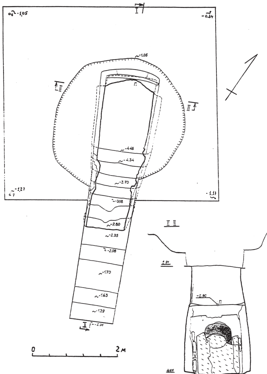
Рис. 4. Некрополь Джург-оба. План розкопу №3 з планом передромосної ями. Розріз по лінії II-II суміщеної з фасом порталу і закладної плити
